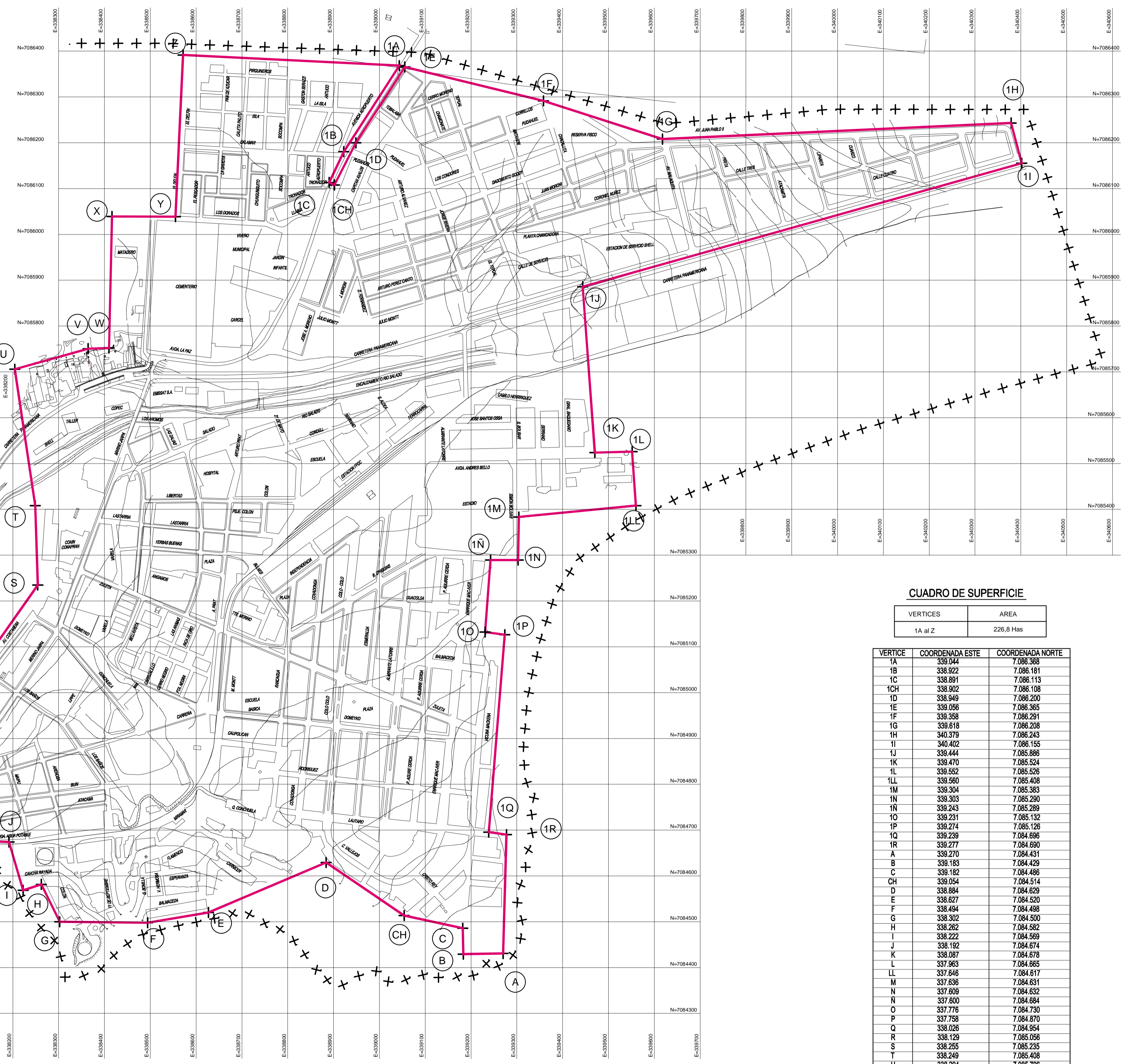
PLANTA GENERAL DE CHAÑARAL TERRITORIO OPERACIONAL ESCALA 1:5.000
